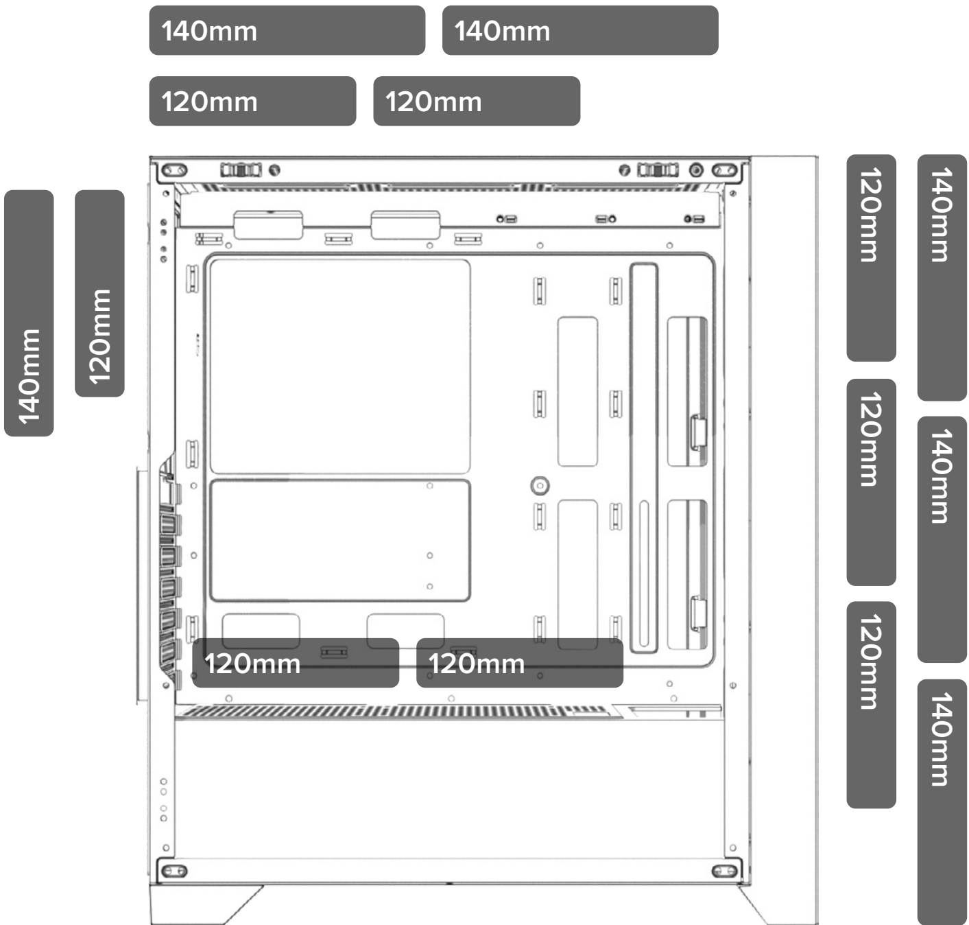
Opciones de instalación de ventiladores
